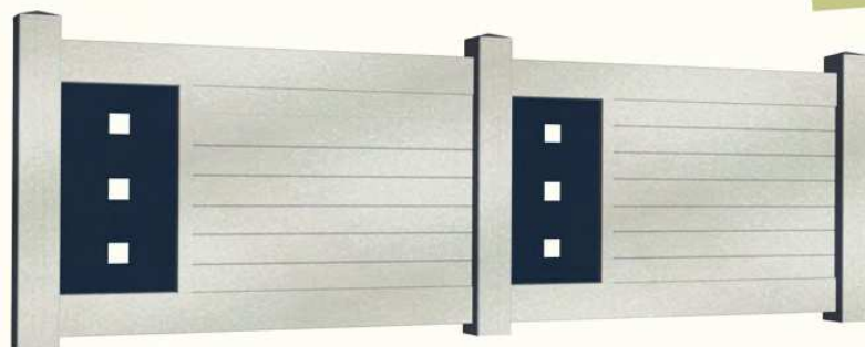
Sagittarius
