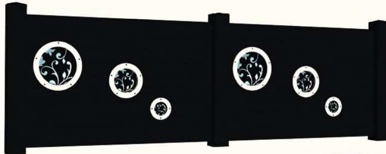
Carina
