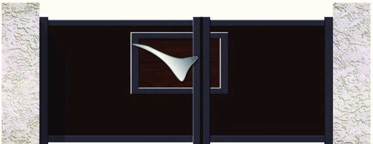
Cetus
