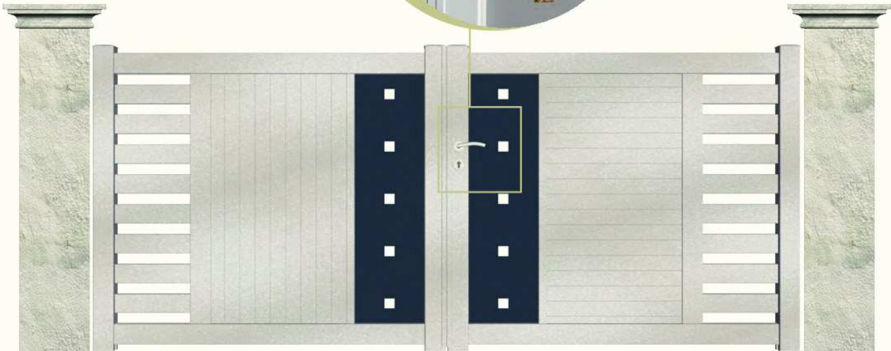
Sagittarius
